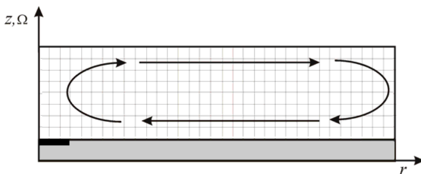
Рис. 1. Схематичное изображение расчетной области и меридиональной циркуляции
